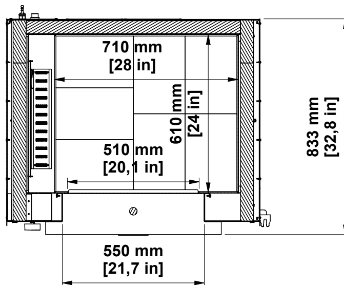
A-A (1 : 15)
