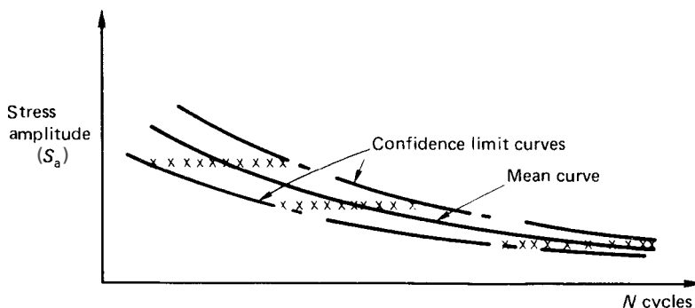
Fig. 15.1 S-N diagram.
