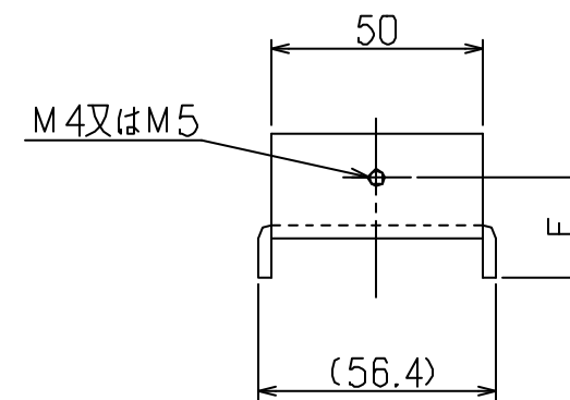
レール取付板参考形状 (S = 1 : 2)
