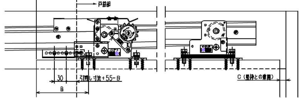
レール、戸当り金具取付用穴位置図(点検口側より見る)
