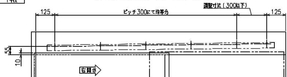
レール取付用穴位置図 (点検口側より見る)
