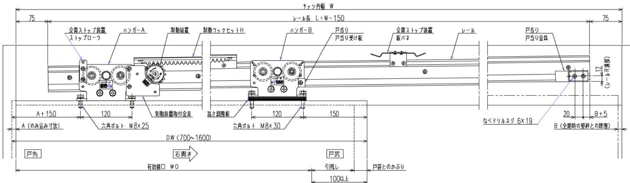
縦断面図 (1:2)
