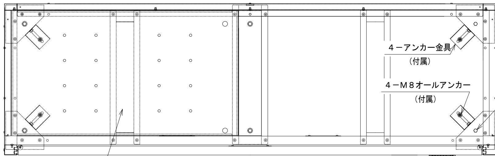
A-A断面図 (右側底板を取り外した状態)
