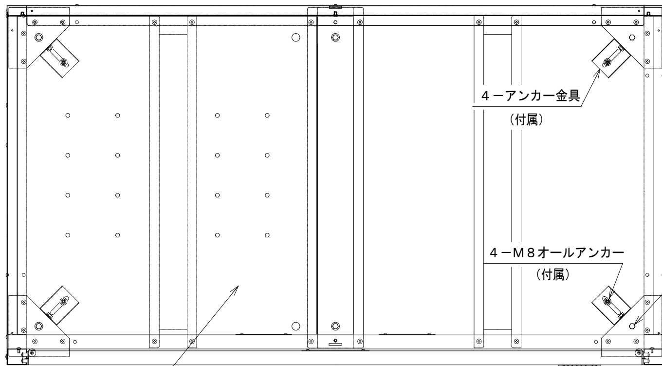
2-底板 (取り外し可能) A-A断面図 (右側底板を取り外した状態) 取手 上扉
