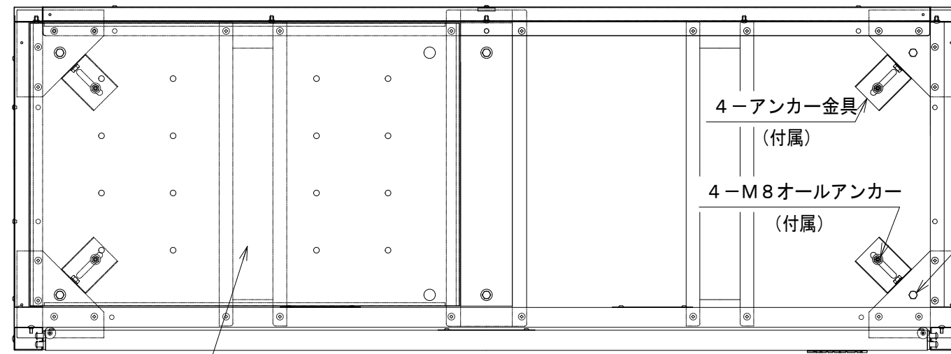
A-A断面図 (右側底板を取り外した状態)
