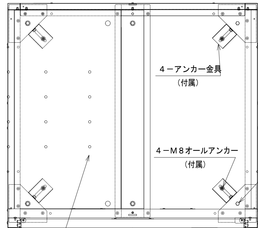
2-底板 (取り外し可能) A-A断面図 (右側底板を取り外した状態)
