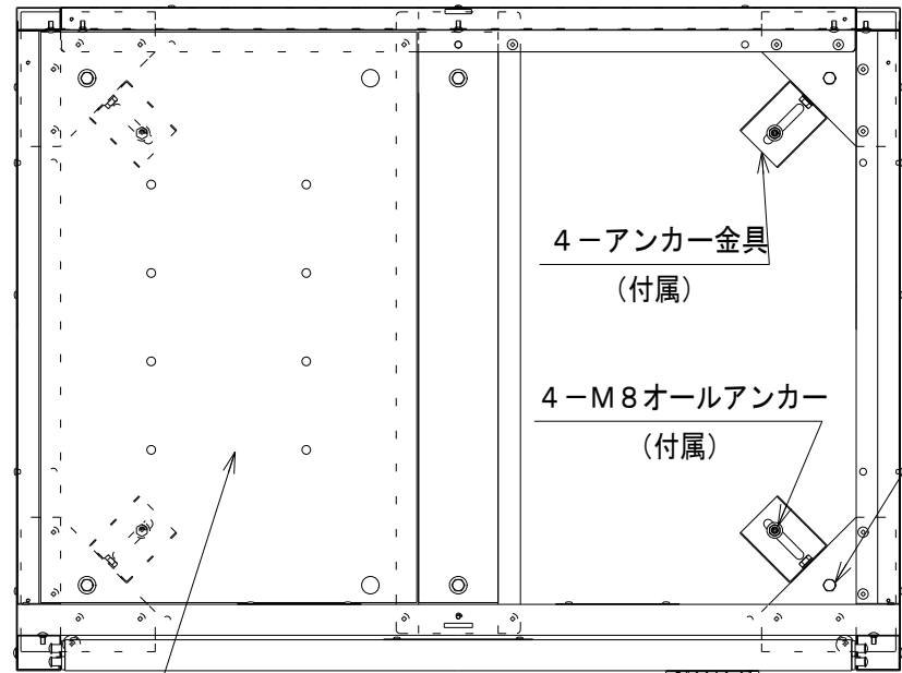
A-A断面図 (右側底板を取り外した状態)
