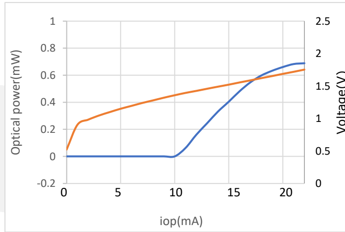
L-I-V Curve
