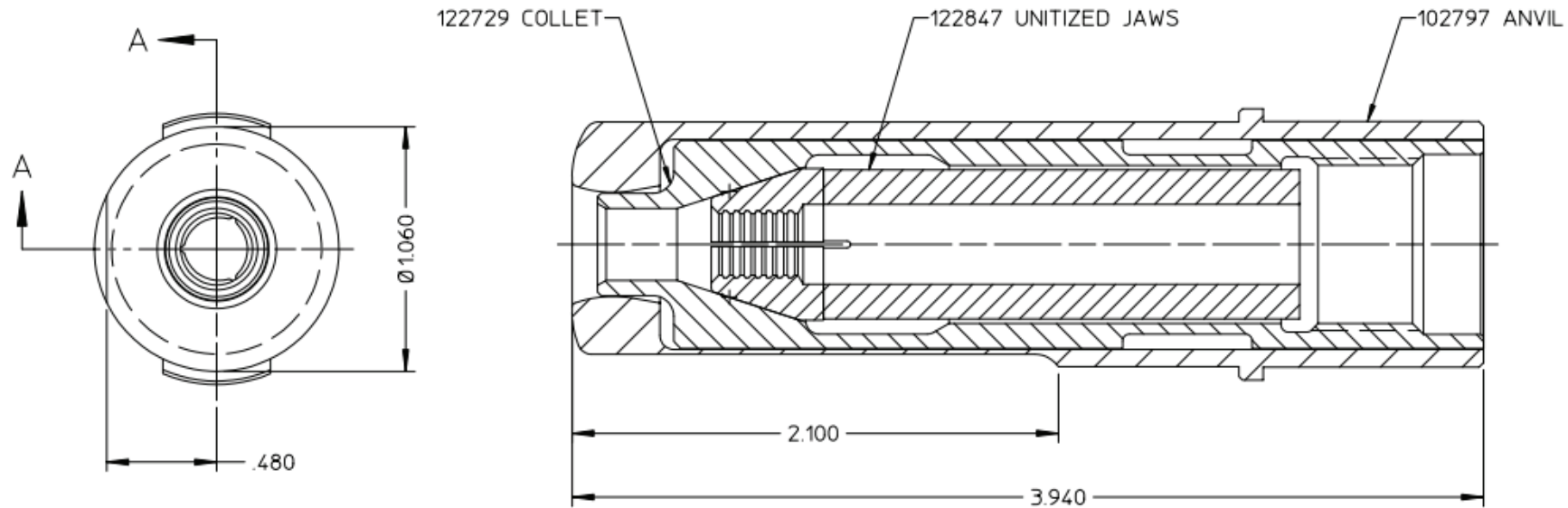
SECTION A-A
