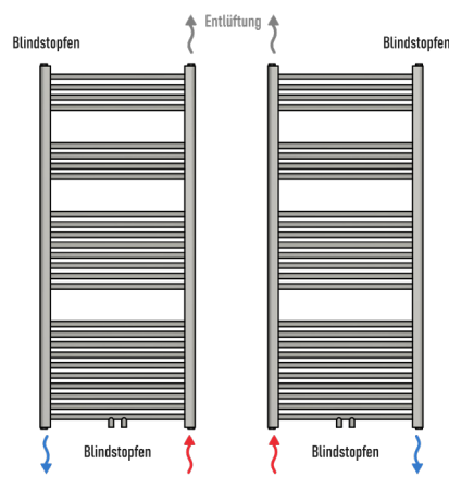
Seitenanschluss
