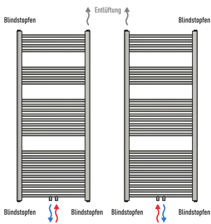
Mittelanschluss
