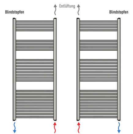
Seitenanschluss
