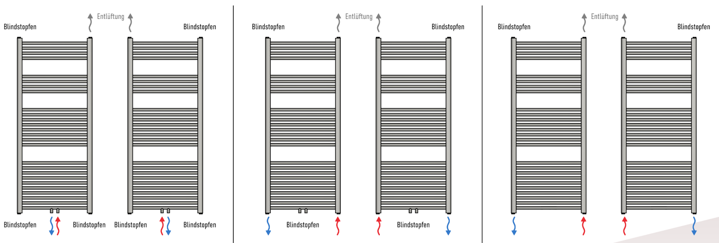
Mittelanschluss
