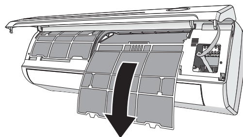
Filtre anti-poussière
