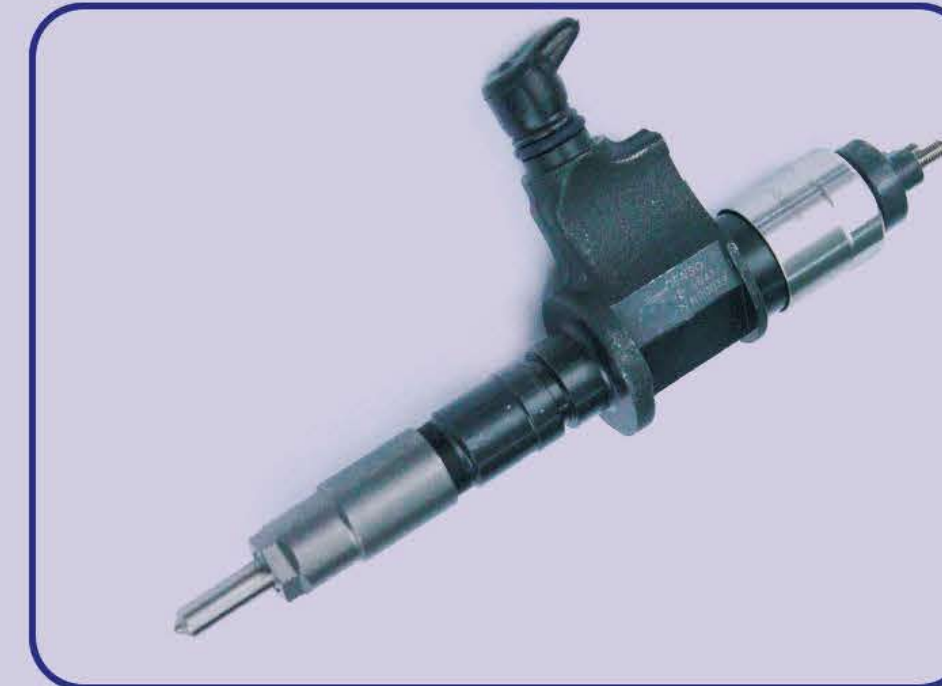
Injector DENSO: 095000-5841
