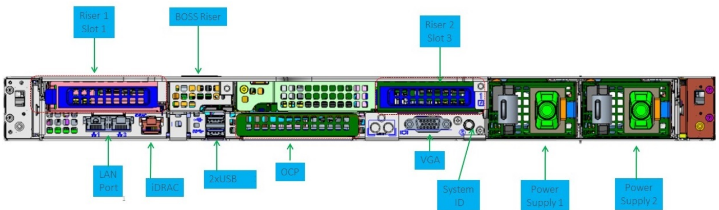
그림 3. 시스템의 후면
