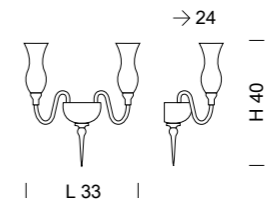
1020/A2 2 x MAX 42W E14
