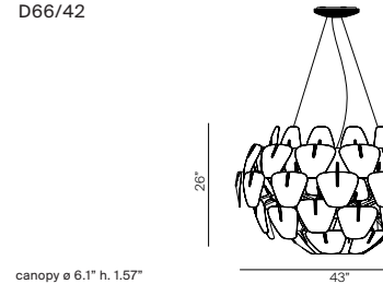
canopy ø 6.1" h. 1.57"
