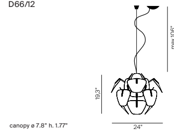
canopy ø 7.8" h. 1.77"
