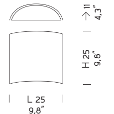
212 2 x MAX 42W E14
