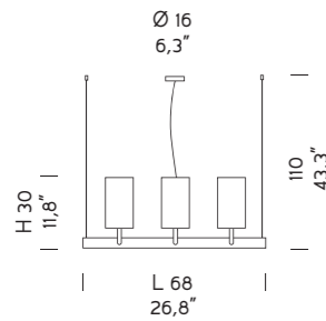
2120/9+3 12 x MAX 42W E14
