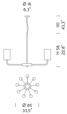
2120/9 9 x MAX 42W E14
