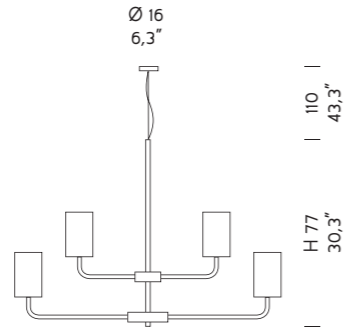
2120/9 9 x MAX 42W E14
