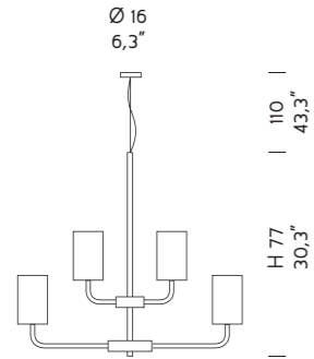
2120/6 6 x MAX 42W E14
