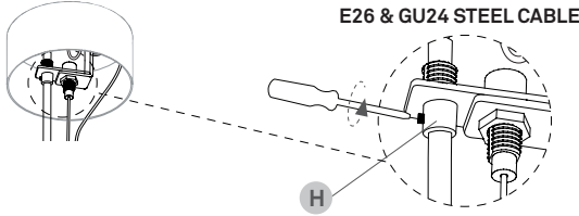
E26 & GU24 STEEL CABLE
