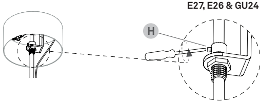
E26 & GU24 STEEL CABLE
