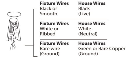
Fig. 2 Wiring
