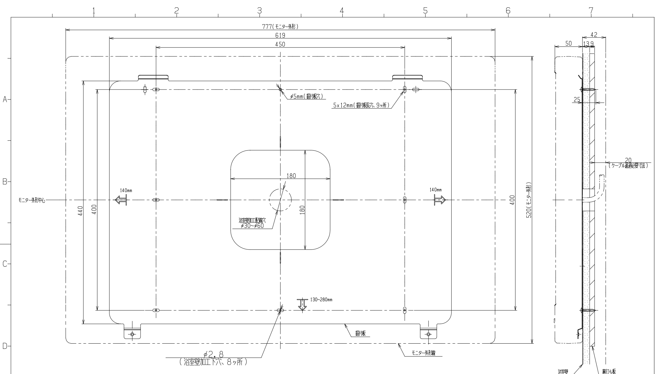
浴室壁加工穴寸法図
