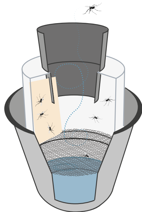
Querschnittsansicht
