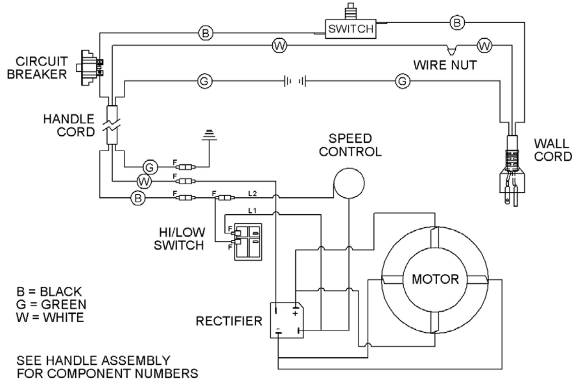
WIRING DIAGRAM - MUSTANG 300 DS - 120 VOLT
