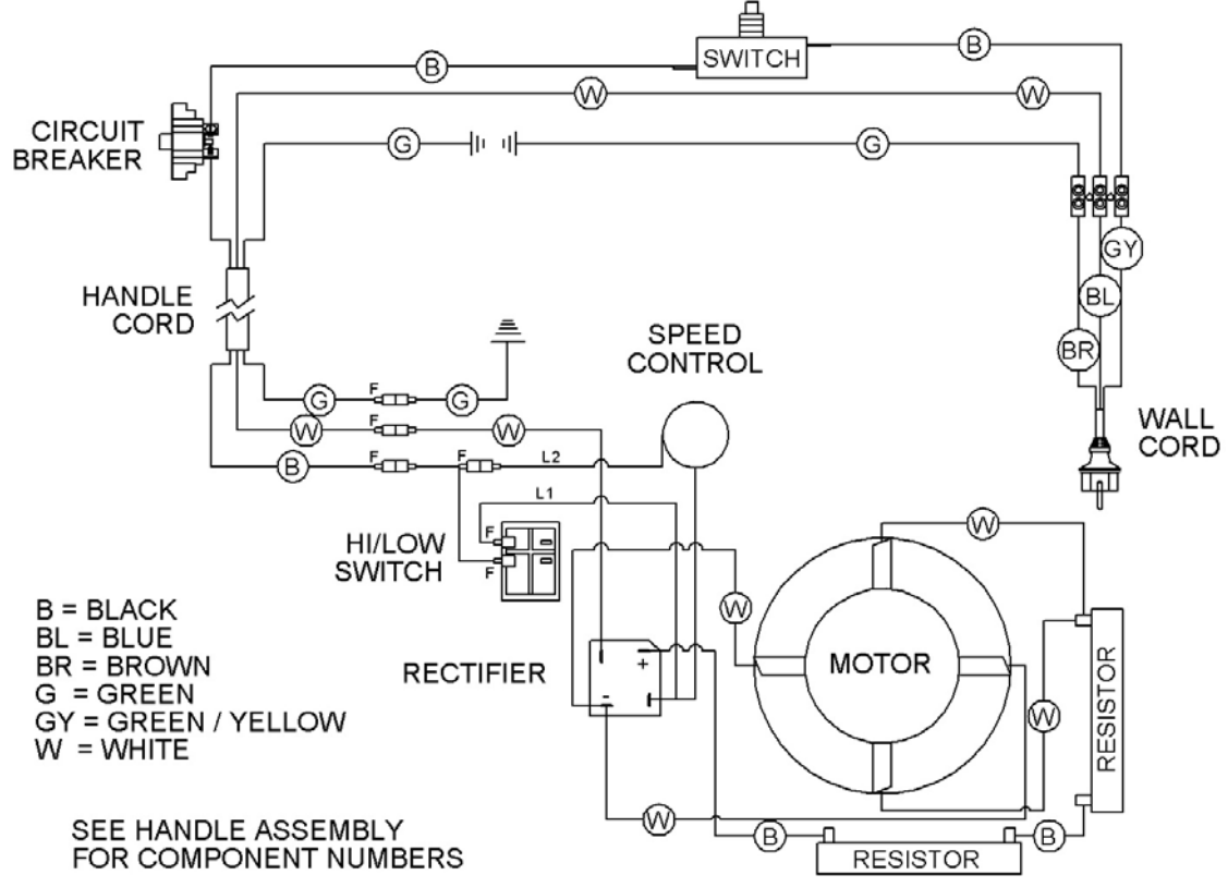
WIRING DIAGRAM - MUSTANG 300 DS - 240 VOLT
