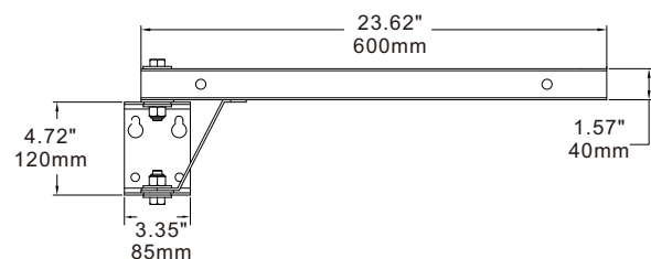
24" Bracket A4
