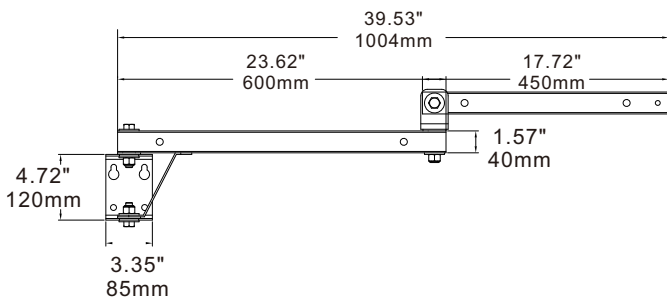
40" Bracket A1
