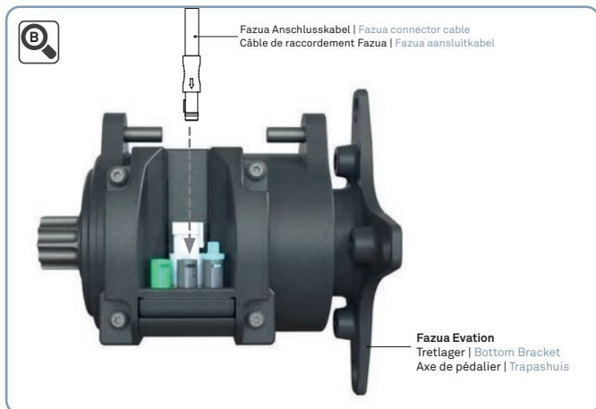
Anschlusskabel Kopplung | Connecting to drive cable Câble de raccordement pour le branchement | Connectie van de aansluitkabel
