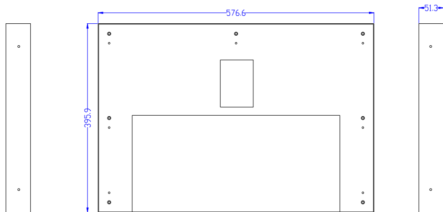
Bracket(Unit:mm)
