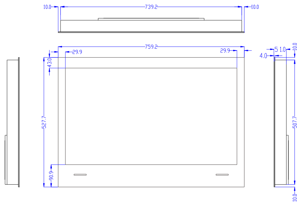
Television(Unit:mm)
