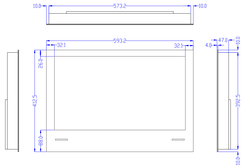
Television(Unit:mm)
