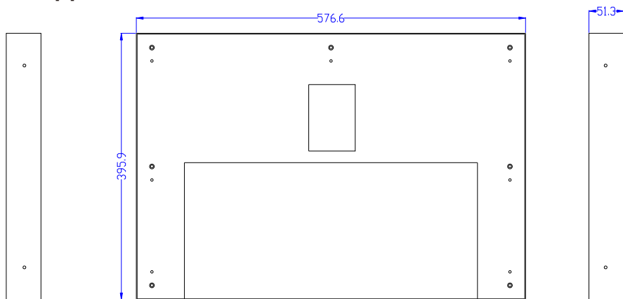
Le support (unité : mm)
