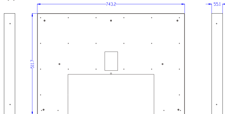
Le support (unité : mm)
