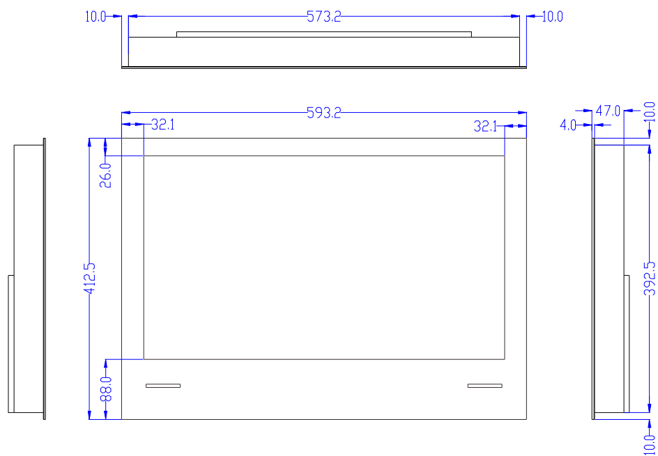
Téléviseur (unité : mm)
