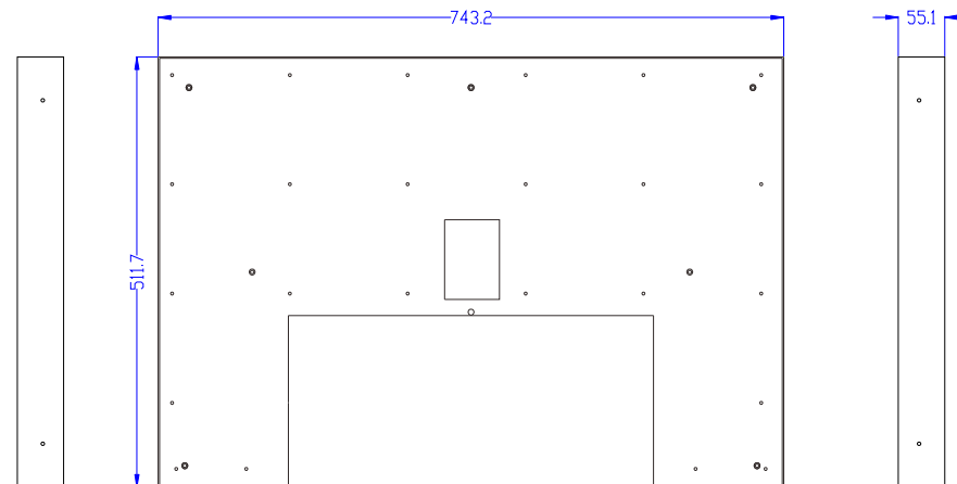
Bracket(Unit:mm)
