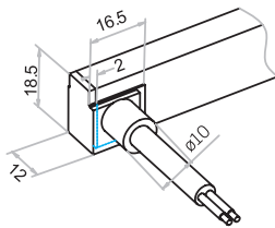
END CAP
