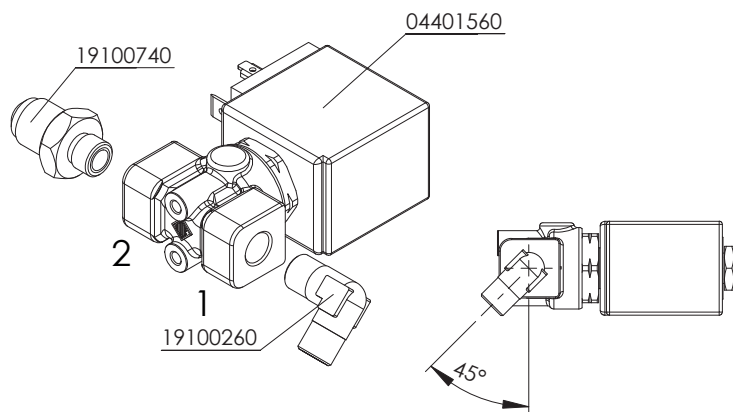
41300060 - FILL SOLENOID BARISTA T ASSEMBLY
