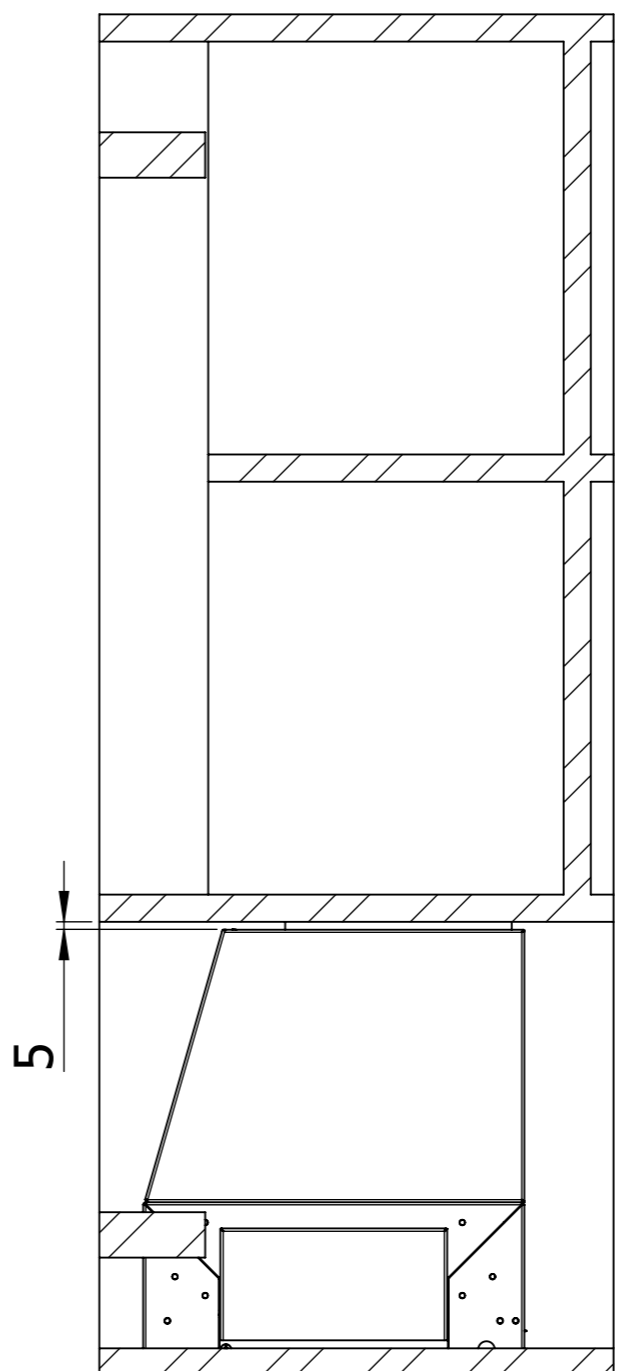
SEZIONE C-C
