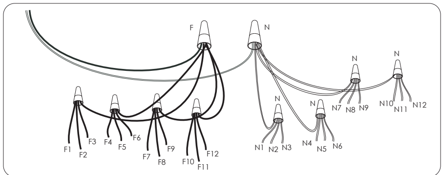
SCHEMA ELETTRICO INTERNO / INTERNAL WIRING DIAGRAM
