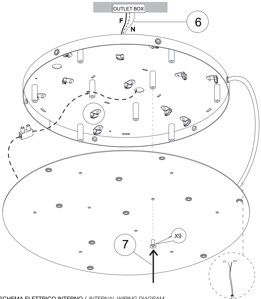
SCHEMA ELETTRICO INTERNO / INTERNAL WIRING DIAGRAM
