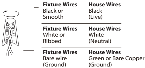
Fig. 3 Wiring
