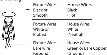
Fig.3 Wiring
