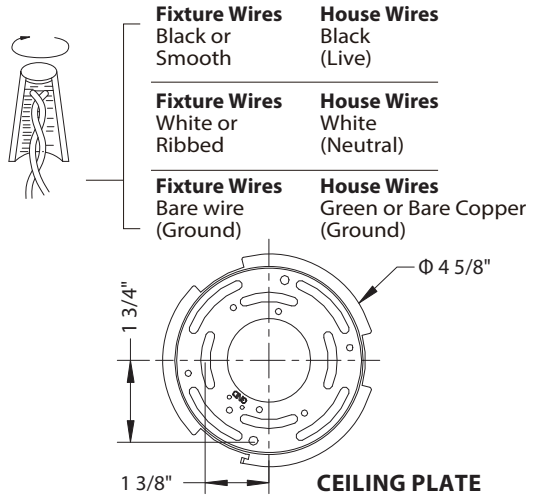
Fig. 2 Wiring
