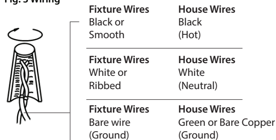
Fig. 3 Wiring
