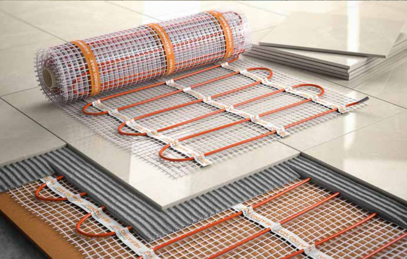
1 Instalar la malla Ecofloor sobre la losa.
