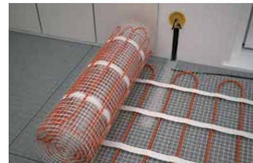
1 Instalar la malla Ecofloor sobre la losa.
