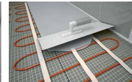
3 Finalmente Instalar piso cerámico o porcelanato.
