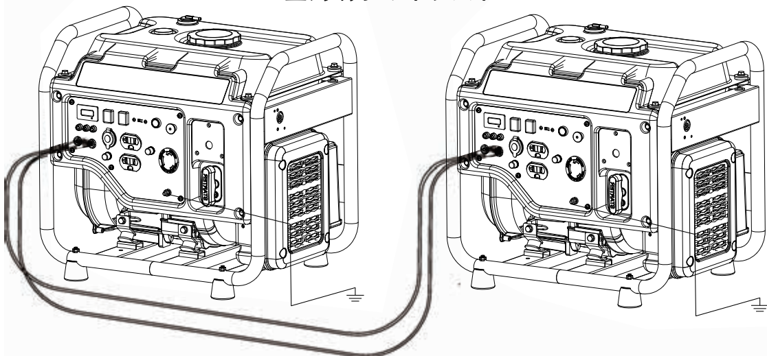
並列端子のイラスト
