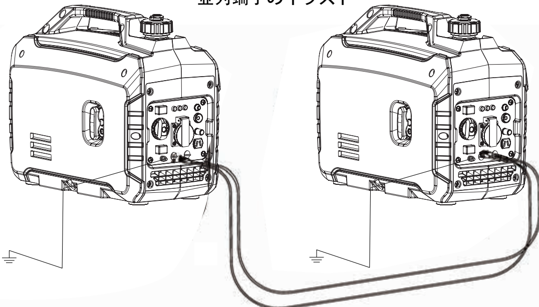
並列端子のイラスト
