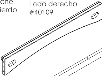
T. Bottom Front Rail x1 Barre avant inférieur Barra frontal inferior #40112
