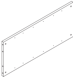
J. Bottom Back Rail x1 Barre arrière inférieur Barra trasero inferior # 29778
