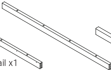
D. Top Front Rail x1 panneau supérieur avant barandilla superior frontal # 28311
