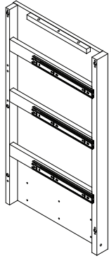
B. Right Side x1 Côté droit Lado derecho #41047
