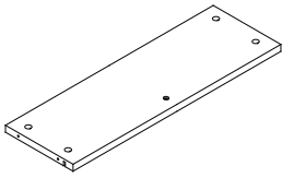
R. Top Drawer Back x2 Arrière du tiroir supérieur Parte posterior de la gaveta superior #41051
