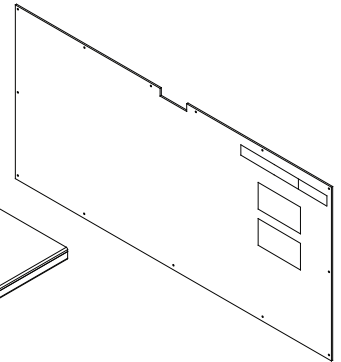
K. Back Panel x1 Panneau arrière Panel trasero #26420
