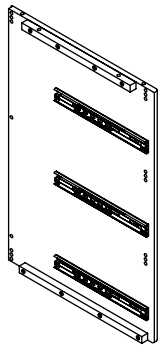
B. Right Side x1 Côté droit Lado derecho # 41030
