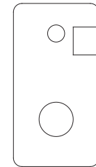
E. Changer Middle Shelf Rail x 2 Traverse de l'étagère centrale de la table à langer x 2 Barra del estante central del cambiador x 2 26453
