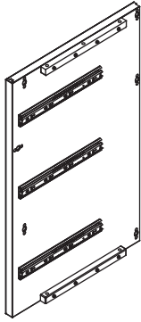
A. Left Side x1 Côté gauche Lado izquierdo #40628
