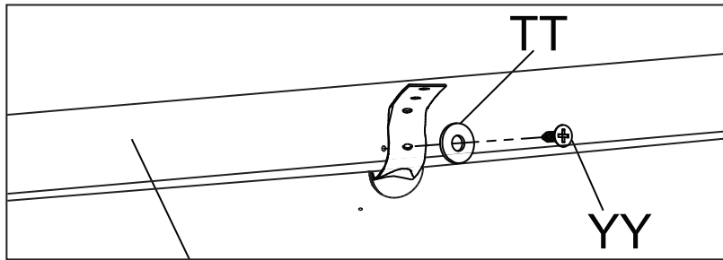
Top Back Rail Barre Arrière Supérieur Barra Trasero Superior
