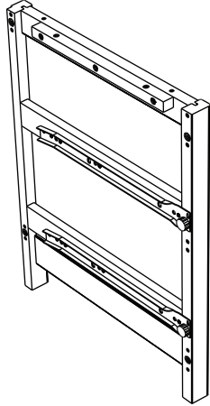
B. Right Side x1 Côté droit Lado derecho # 29332
